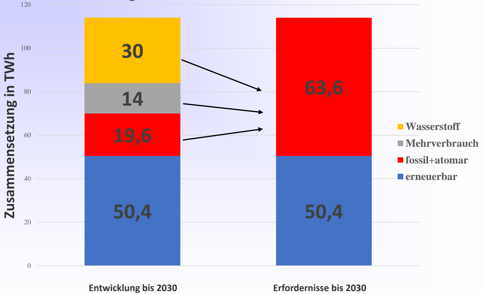
Entwicklung des Stromverbrauchs in TWh bis 2030
